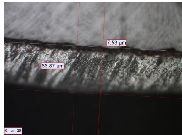
Bild: Schichtaufbau, Stahl-Hartzink-Zinklegierung
